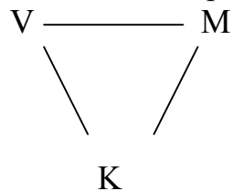
Leibliches Ursprungsdreieck
