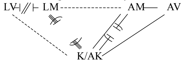
Adoptionsdreieckssystem
